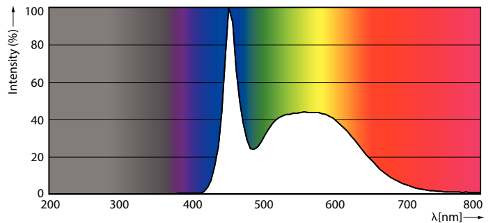
LEDtube_18W_G13_2100lm_865
